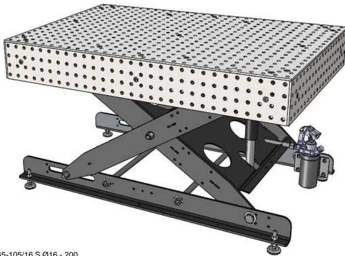
Bild : 3D Modell SWT 65-105/16 S Ø16 - 200
